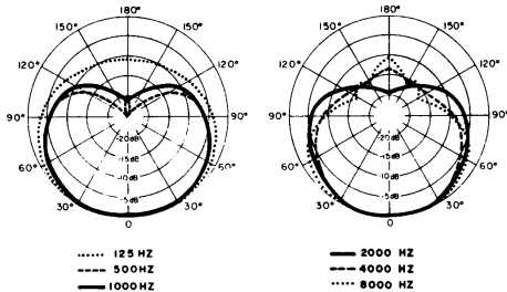
COURBES DE DIRECTIVITÉ TYPQUES FIGURE 3
