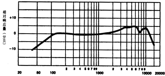
典型频率响应 图 2
